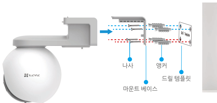
그림 2 벽 장착
