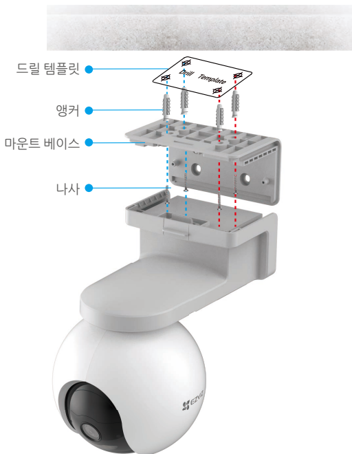
그림 1 천장 장착
